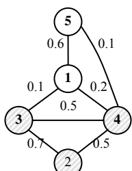
Fig.4 The initial graph for BestCut 图 4 BestCut 方法中的初始图
