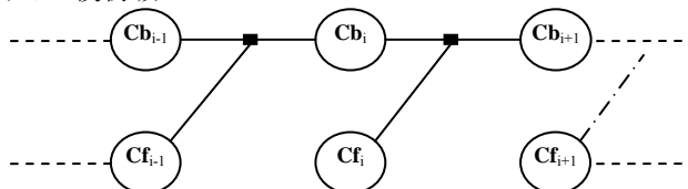
Fig.6 Coreference resolution model based on centering theory and CRF 图 6 基于中心理论和 CRF 的共指消解模型
